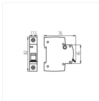
KMB6-B20/1
