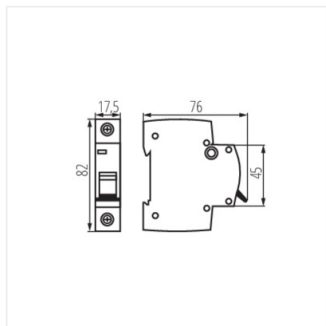
KMB6-B25/1
