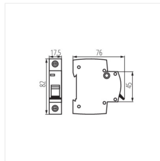
KMB6-B32/1
