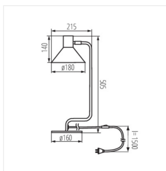
NEDIA E14 W
