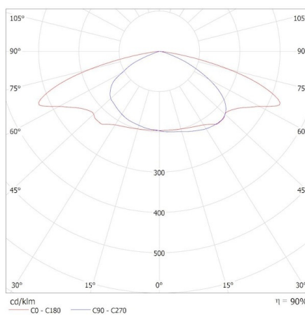
KANLUX S.A. (kat 39300) PRO-S S 65W-ZH NW / Krzywa rozsyłu światła (biegunowo)
