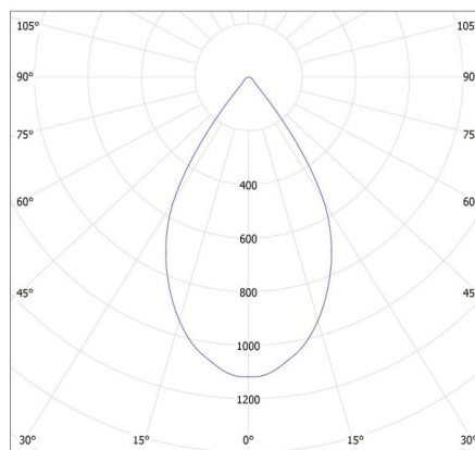
KANLUX S.A. (kat 33134) ATL1 30W-930-S6-W / LDC (Polar)
