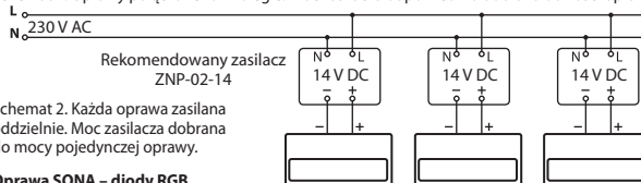
Schemat 2. Każda oprawa zasilana oddzielnie. Moc zasilacza dobrana do mocy pojedynczej oprawy.
